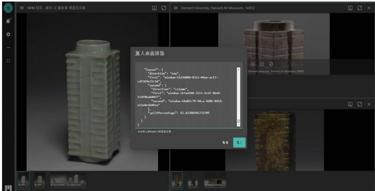
圖14 匯入時，點選「匯入桌面排版」，將上次匯出儲存的系統程式碼複製貼上，就可以從上次的排版開始使用。
